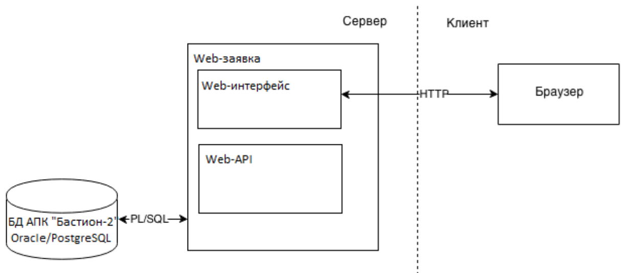
Рис. 1 Структура системы "Бастион-2 – Web-заявка"
